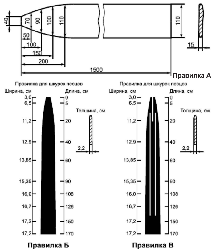
Рисунок. Правилки для правки шкурок песка мездрой (А) и волосом (Б, В) наружу Figure. Frames for straightening arctic fox skins with a mezdra (A) and a hair (Б, В) out
